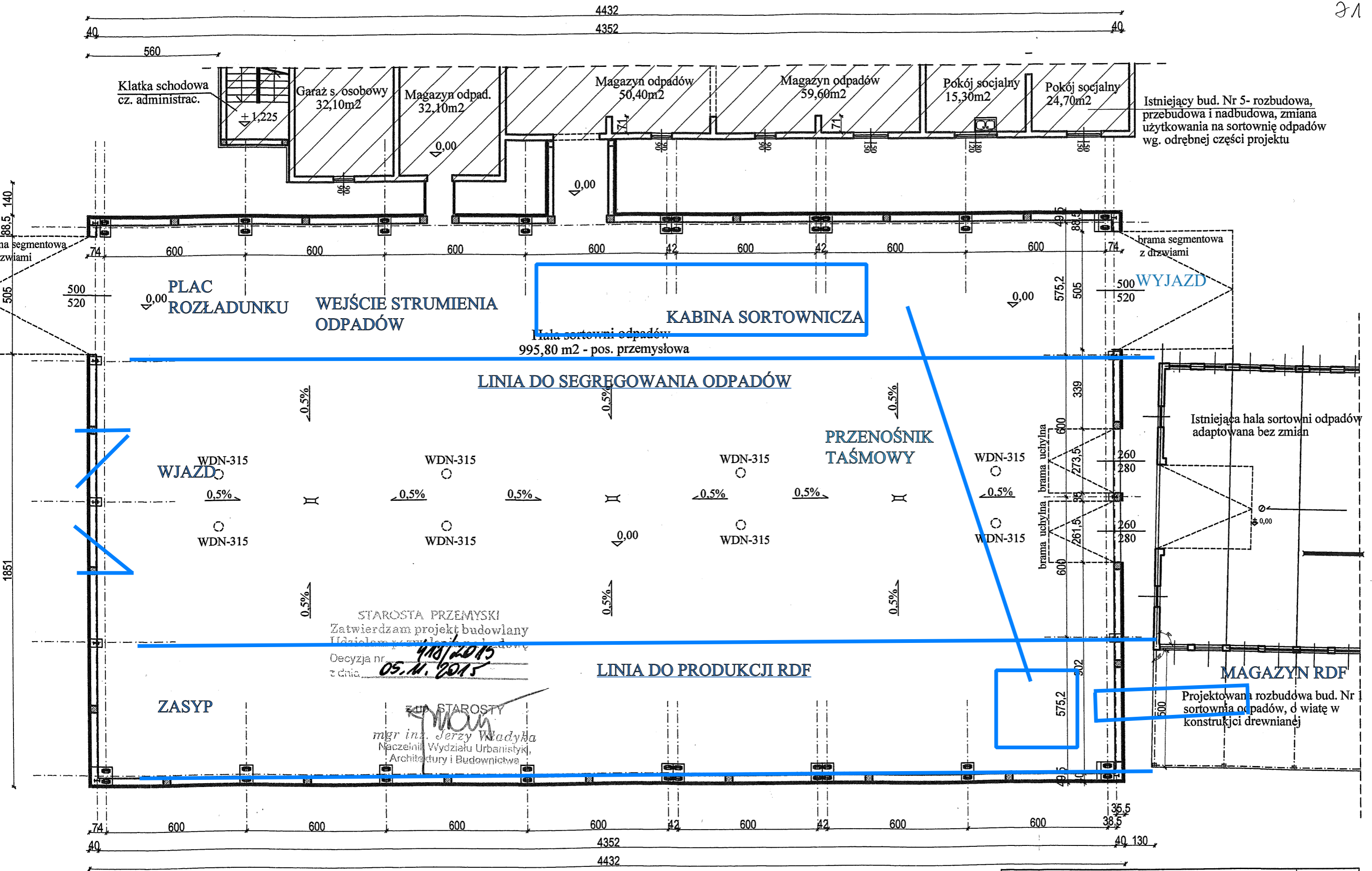
Rzut przyziemia - Hala sortowni odpadów 1 : 150
